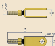
PONTEIRA GARFO CIL DE 2.1/2 3T (A) 12,8MM (B) 97MM (C) 28MM (D) 17MM
